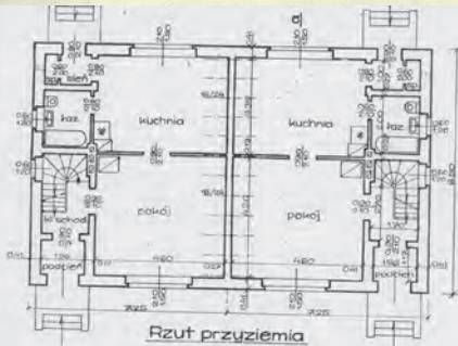
Rzut przziemia
