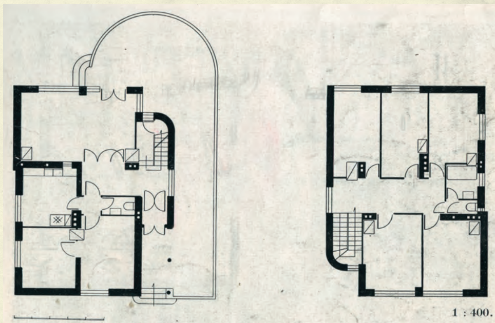
Rzuty poziome parteru i piętra domu im. Ignacego Boenera przy ul. Ignacego Boenera nr 5. Projektował inż. arch. Jan Reda
