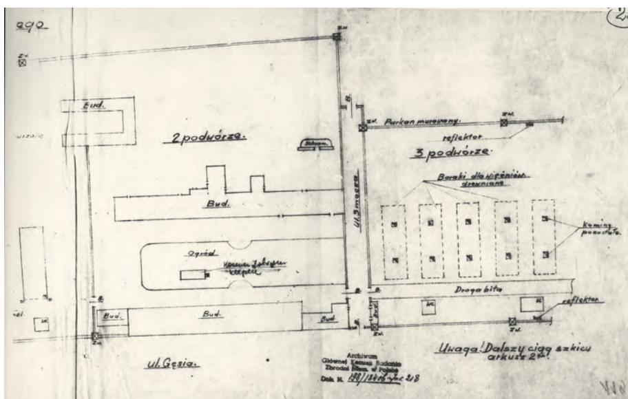
14. Szkic sytuacyjny terenu byłego obozu koncentracyjnego Warschau z 20 maja 1946 r., wykonany przez kaprała MO Stanisława Staszczyka.
